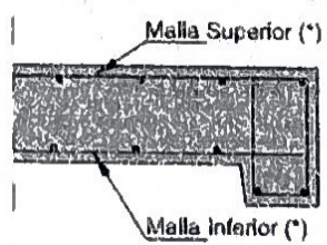
ARMADURA DE LOSA DE TAPA
