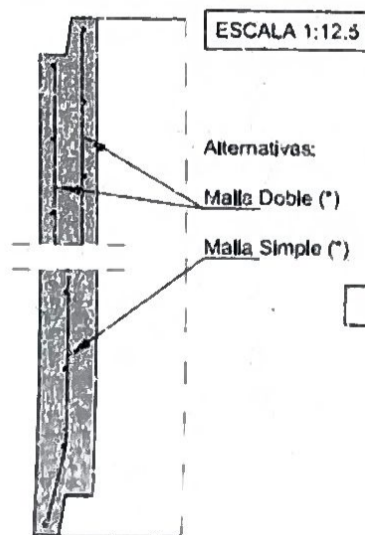
ARMADURA DE PARED DE CUERPO
