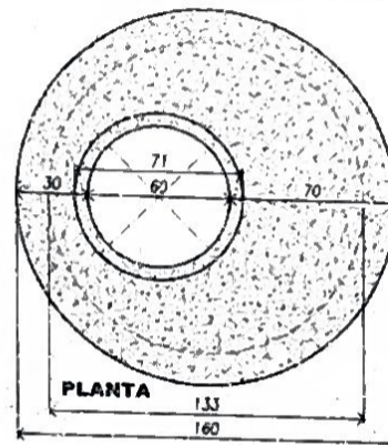
LOSA DE TAPA CON ABERTURA DE ACCESO
