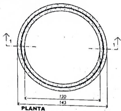
MÓDULO CUERPO DE CÁMARA Ø120
