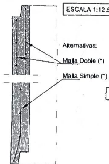
ARMADURA DE PARED DE CUERPO
