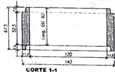
MÓDULO Ø120 - L = 60 cm
